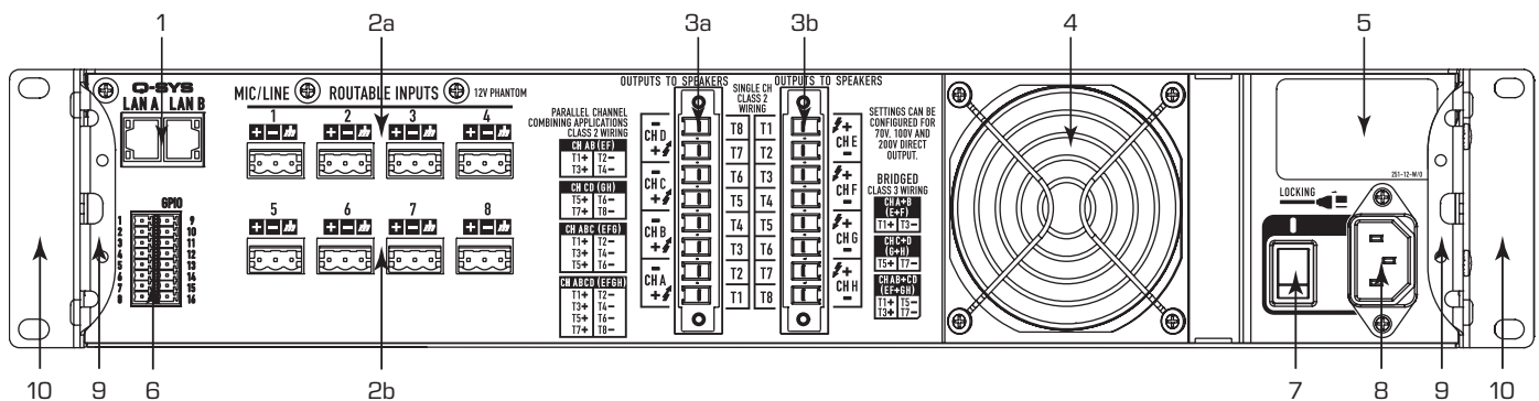
— 图 1 — CX-Q 显示的八通道型号
