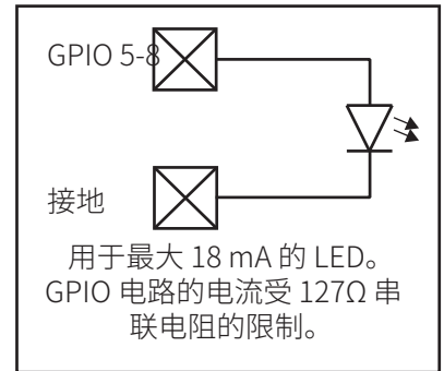
Q-SYS提供电源的LED
